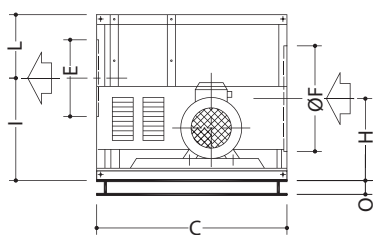
CCT - Quote principali con motori da 11 kW e oltre
