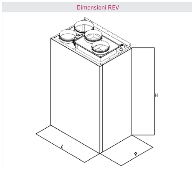
DIMENSIONI REV (mm)
